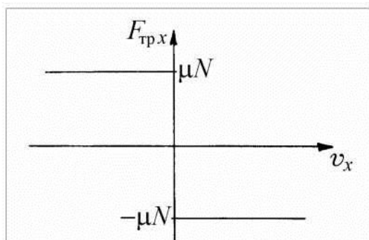
Рис. 4.2. Сухое трение
