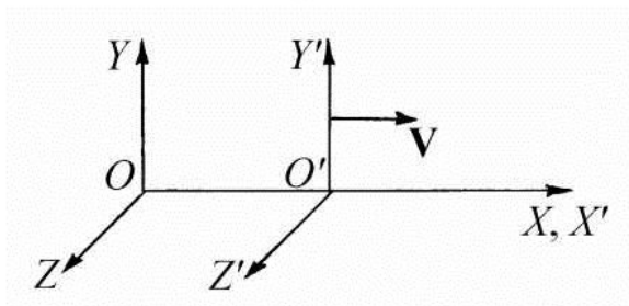
Рис. 6.1. Неподвижная и движущаяся системы отсчета
