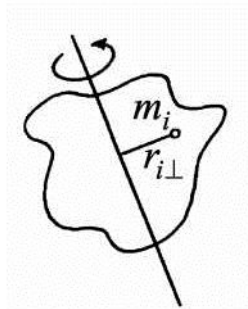
Рис. 8.1 К вычислению момента инерции
