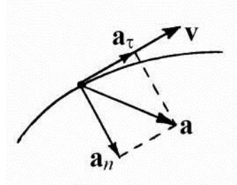
Рис. 1.5. Тангенциальное и нормальное ускорения
