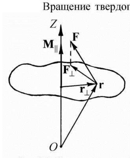
Рис. 9.1. К вычислению момента силы
