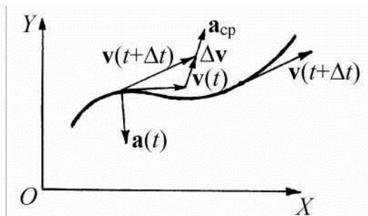
Рис. 1.4. Среднее и мгновенное ускорения
