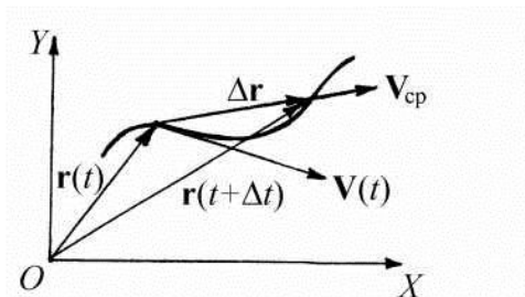
Рис. 1.3. Средняя и мгновенная скорости
