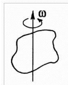
Рис. 10.2. К вычислению момента импульса тела с неподвижной осью вращения
