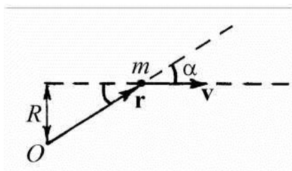
Рис. 10.1. К вычислению момента импульса материальной точки
