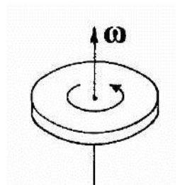
Рис. 2.1. Вектор угловой скорости
