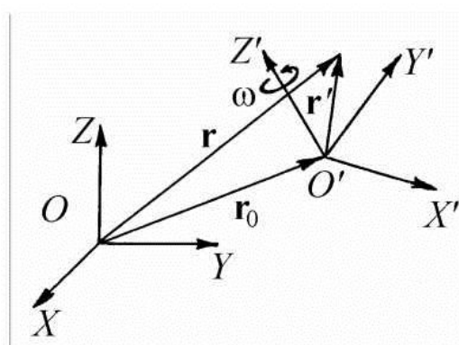
Рис. 3.16. Неподвижная и движущаяся системы отсчета
