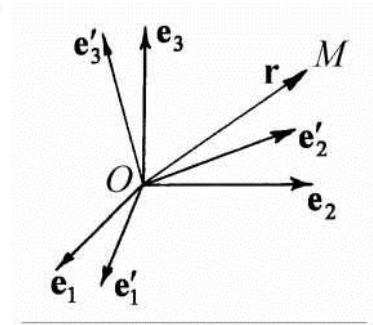
Рис. 2.2. К выводу матрицы поворота
