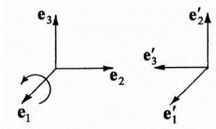
Рис. 2.3. Поворот вокруг оси x_1 на 90^\circ
