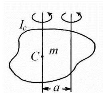
Рис. 8.2 К теореме Гюйгенса-Штейнера
