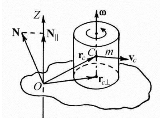
Рис. 10.3. Плоское движение твердого тела
