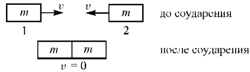
Рис. 6.3. Неупругое соударение двух равных масс.
