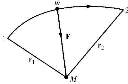
Рис. 7.7. Работа силы гравитационного притяжения двух точечных масс.
