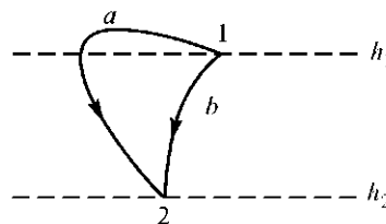
Рис. 7.4. То же, что и на предыдущем рисунке, но в случае криволинейной траектории частицы.
