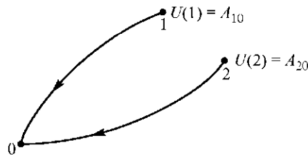
Рис. 8.1. Определение потенциальной энергии.
