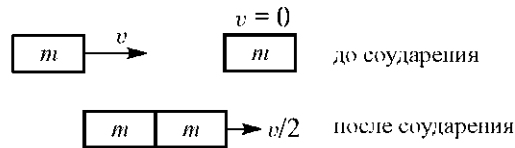
Рис. 6.5. Неупругое соударение двух равных масс, одна из которых покоится, — итог.
