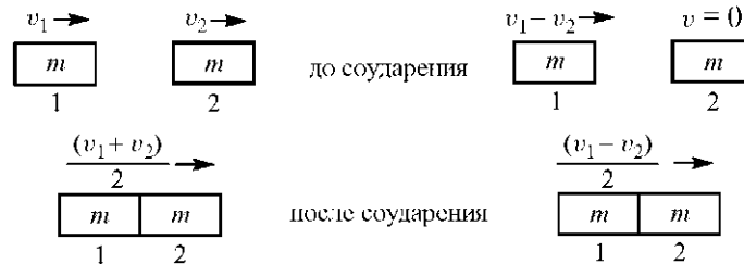
Рис. 6.6. Неупругое соударение двух равных масс, движущихся с произвольной скоростью. Слева — лабораторная система отсчета, справа — система отсчета, связанная с одной из масс.
