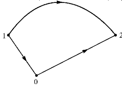
Рис. 8.3. Работа консервативных сил равна убыли потенциальной энергии системы.
