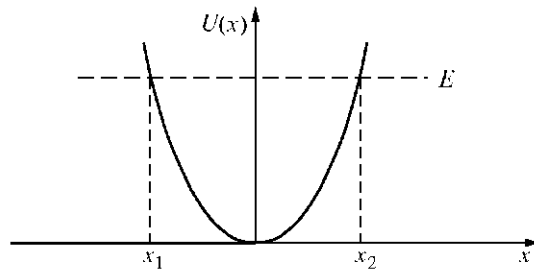
Рис. 8.9. Движение в квадратичном потенциале. Гармонические колебания.
