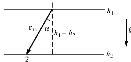
Рис. 7.3. Работа силы тяжести зависит только от разности высот h_1 - h_2 .
