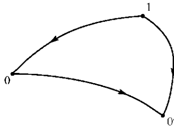
Рис. 8.2. Потенциальная энергия зависит от выбора нулевого положения.
