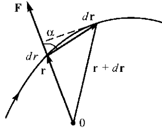
Рис. 7.6. Работа центральных сил.
