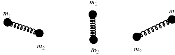
Рис. 6.1. Свободное движение двух тел, связанных пружинкой.
