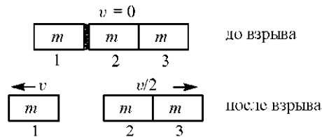
Рис. 6.8. Разлет тел массы m и массы 2m .
