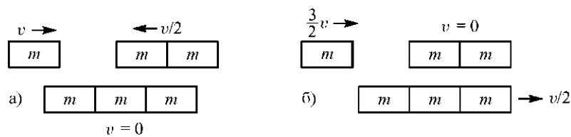
Рис. 6.9. а) Неупругое столкновение двух тел с массами m и 2m . б) То же самое, но в системе отсчета, в которой тело массы 2m покоится.
