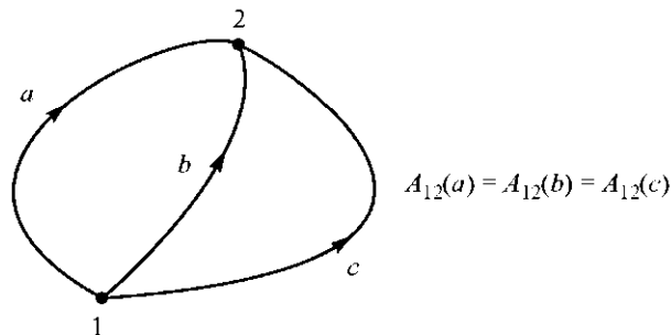
Рис. 7.2. Работа консервативной силы не зависит от пути перехода.
