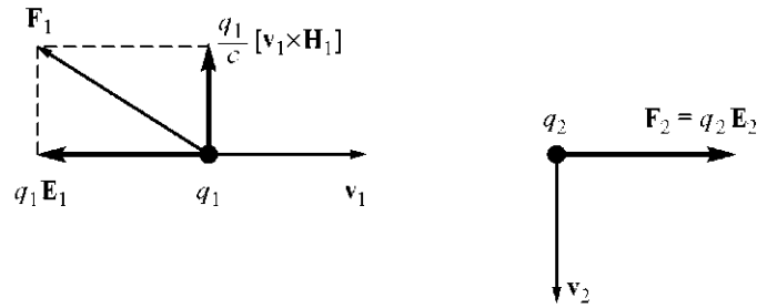
Рис. 5.1. Силы взаимодействия между двумя движущимися зарядами не всегда равны и противоположны.
