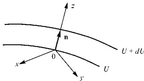
Рис. 8.5. Геометрический смысл градиента ( dU > 0 ).
