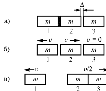
Рис. 6.7. Три одинаковых массы: а) ситуация до взрыва, б) через очень короткое время после взрыва, в) спустя некоторое время после взрыва.
