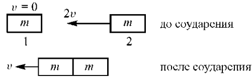
Рис. 6.4. Неупругое соударение двух равных масс в системе отсчета одной из них.
