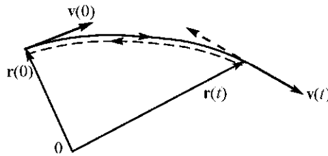
Рис. 7.11. Обращение движения вспять. Частица пойдет назад по той же самой траектории!
