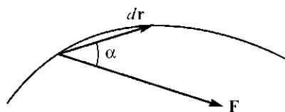
Рис. 7.1. Работа равна скалярному произведению силы на перемещение.
