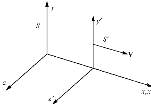
Рис. 5.2. Две инерциальные системы отсчета.
