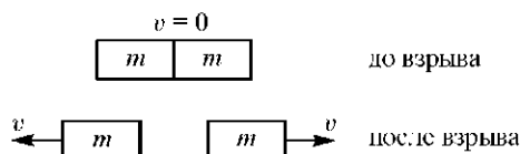
Рис. 6.2. Разлет двух равных масс в результате взрыва.
