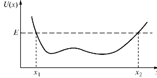
Рис. 8.8. Периодическое движение.
