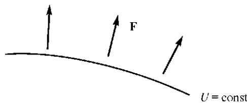
Рис. 8.6. Семейство силовых линий и эквипотенциальных поверхностей взаимно ортогональны друг другу.
