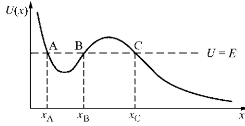
Рис. 8.7. Границы движения в одномерном случае.
