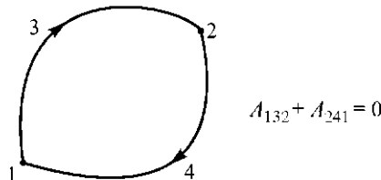
Рис. 7.8. Работа консервативных сил на замкнутом контуре равна нулю.
