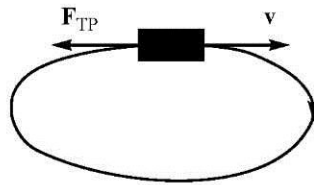
Рис. 7.10. Работа силы трения на замкнутом контуре не равна нулю.
